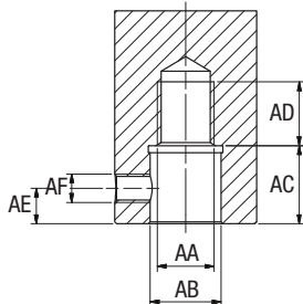
Connessione stelo
